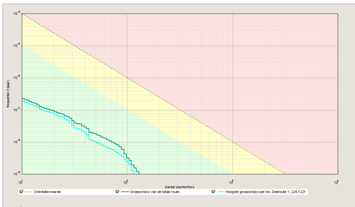
Figuur 3.1: Voorbeeld f/N curve
