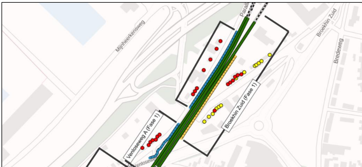
Figuur 7-3 Saneringsmaatregelen Roermond (groen zijn raildempers, blauw is 1m hoog scherm en geel is 3m hoog scherm)
