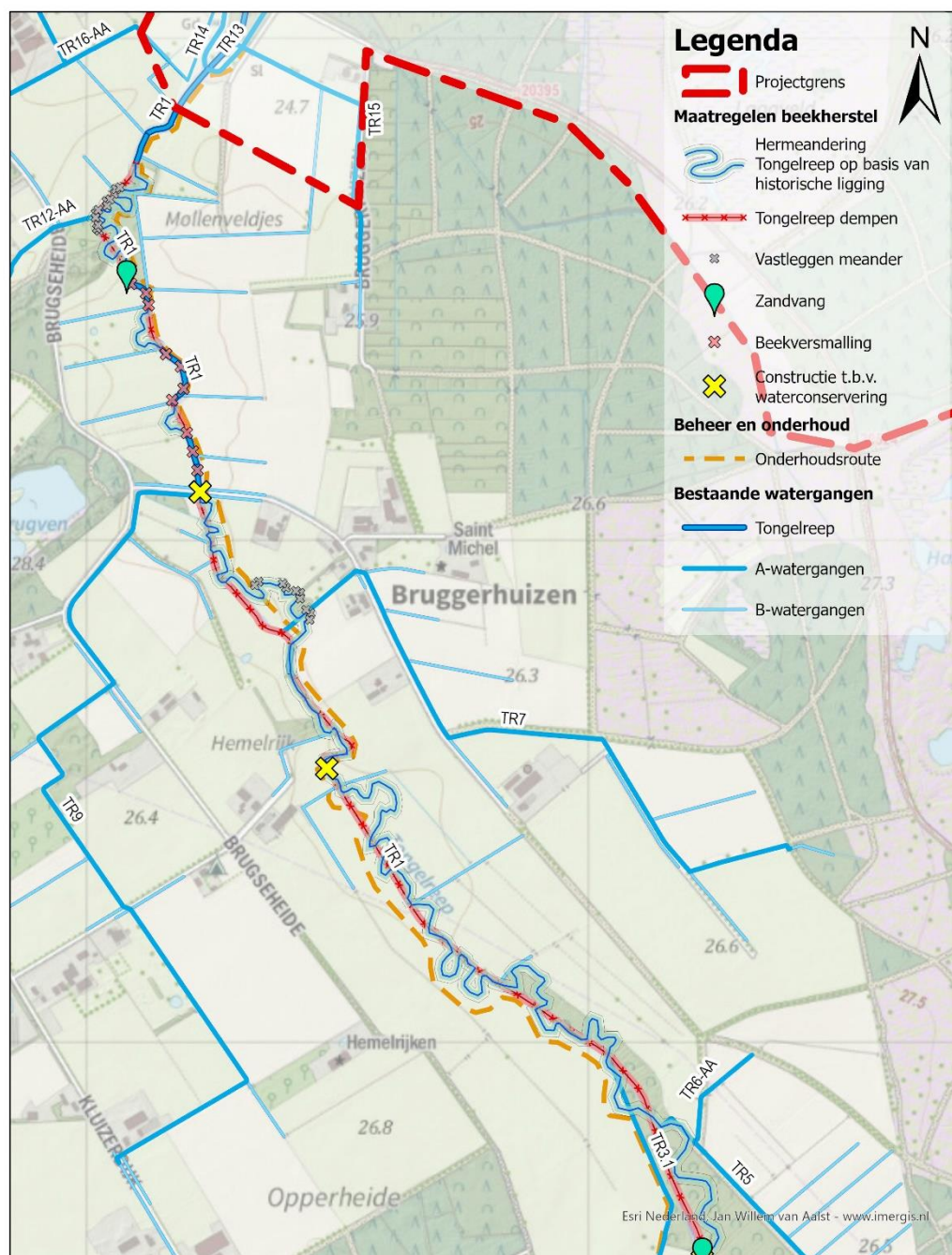
Figuur 1.5-2 Beekherstel met hermeandering Tongelreep op traject 3
