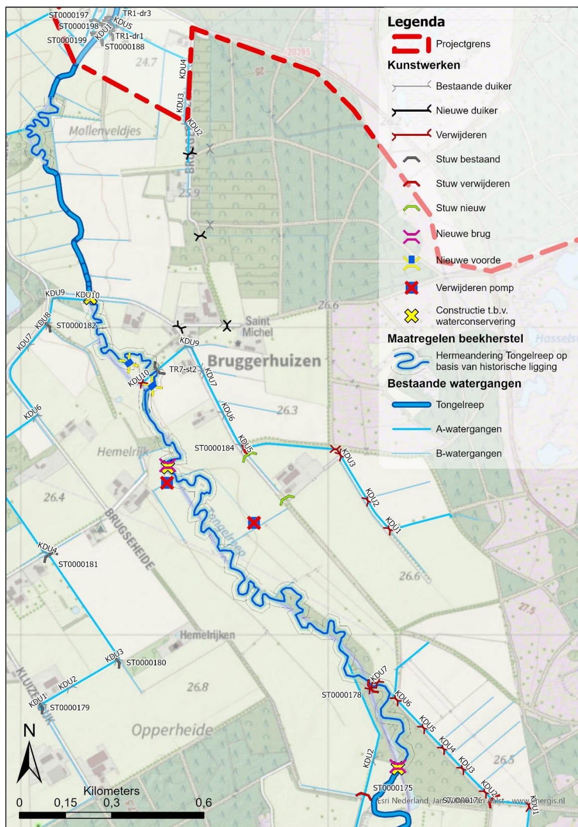
Figuur 1.5-10 Overzichtskaartje met maatregelen kunstwerken rondom traject 3
