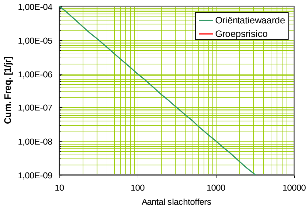
Afbeelding 3: Uitkomst groepsrisicoberekening [4]
