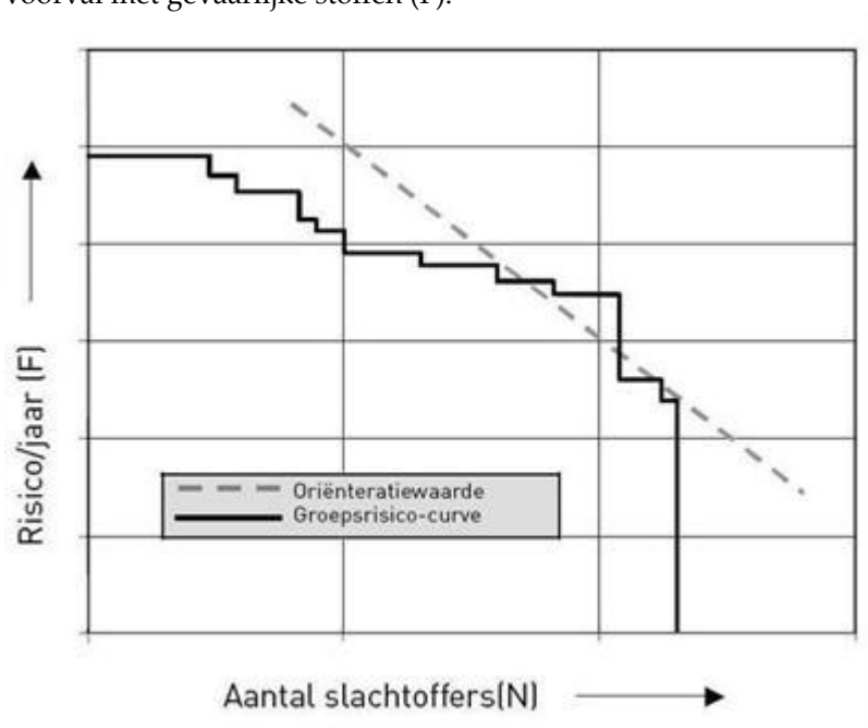
Afbeelding 1: voorbeeld fN-curve
